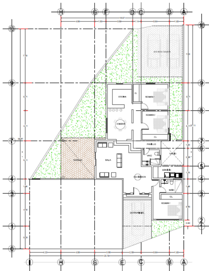
PLANTA ARQUITECTONICA EN UN NIVEL
