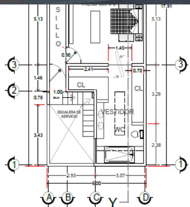
PLANTA ARQUITECTÓNICA ALTA METROS DE CONSTR. 95.65 M2
