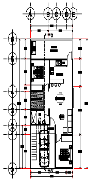
PLANTA ARQUITECTONICA
