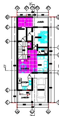
PLANTA ARQUITECTONICA BAJA ESCALA 1:100
