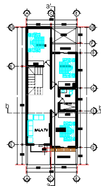
PLANTA ARQUITECTONICA ALTA ESCALA 1:100
